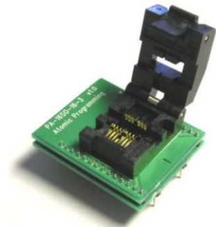
SOIC adapter
